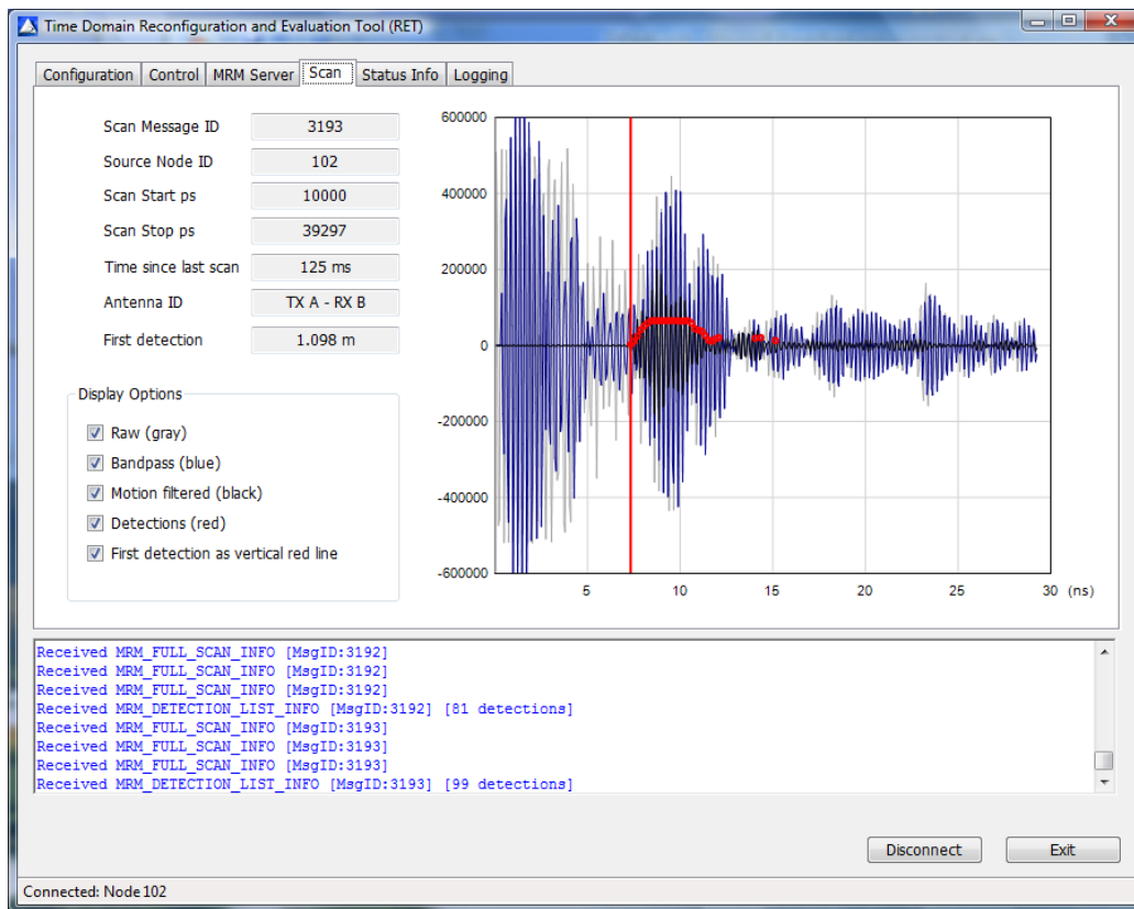
Fig. 8: Scan Tab
