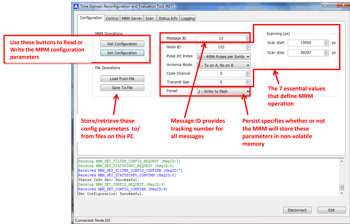
Fig. 4: Configuration Tab
